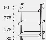
RGM 080V 01 BHT 300 - 600 x 800 x 200
