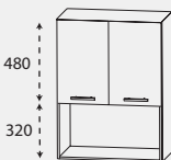
RV 51V 01 / RV 51V T1 BHT 150 - 600 x 800 x 150 - 300 BHT 150 - 600 x 800 x 301 - 470
