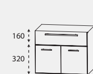
RV 43V 01 / RV 43V T1 BHT 150 - 600 x 560 x 150 - 300 BHT 150 - 600 x 560 x 301 - 470
