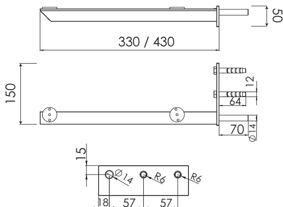
Konsole für Waschtischplatten PZ 1244 50/40
