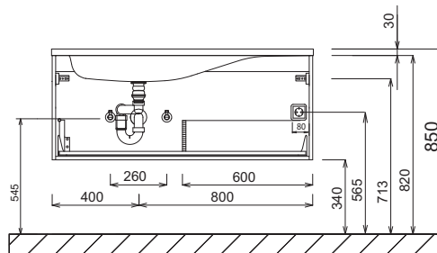
Lavabo simple droit 1200 mm hauteur du lavabo correspond à la hauteur du lavabo Stoneplus
