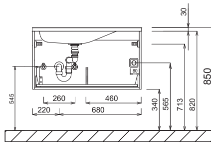
Lavabo simple droit 900 mm hauteur du lavabo correspond à la hauteur du lavabo Stoneplus
