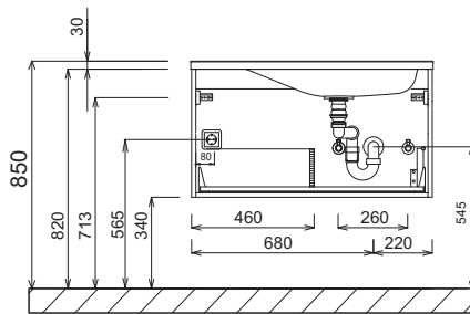
Lavabo simple gauche 900 mm hauteur du lavabo correspond à la hauteur du lavabo Stoneplus
