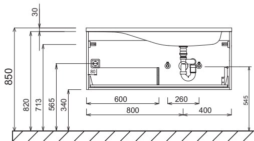
Lavabo simple gauche 1200 mm hauteur du lavabo correspond à la hauteur du lavabo Stoneplus
