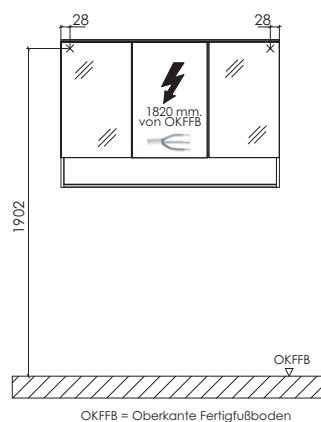
Elektroanschlüsse für Spiegelemente
