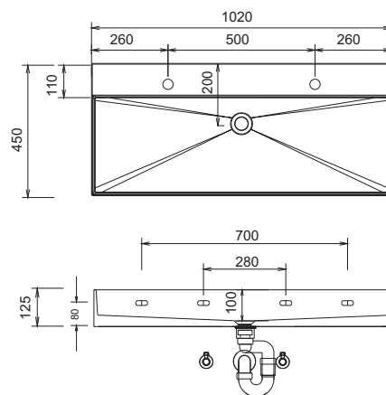
WTM 4821 1 / WTO 4810 1 Schets met kraangat
