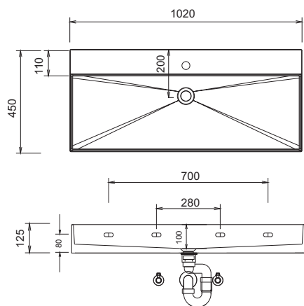
WTM 4810 1 / WTO 4810 1 Schets met kraangat
