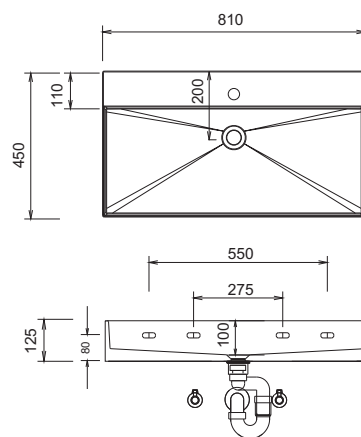
WTM 4808 1 / WTO 4808 1 Schets met kraangat
