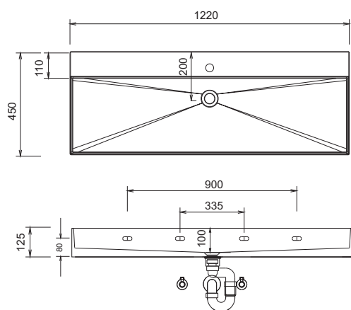
WTM 4812 1 / WTO 4812 1 Schets met kraangat
