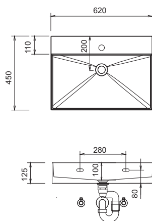
WTM 4806 1 / WTO 4806 1 Schets met kraangat
