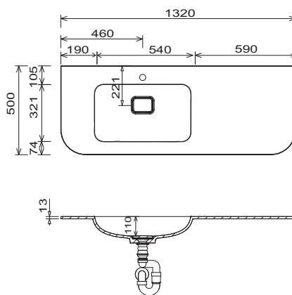
Möbelwaschtisch WMS 263R 61
