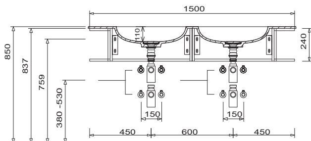
Doppelwaschtisch Unterschrankhöhe 240 mm
