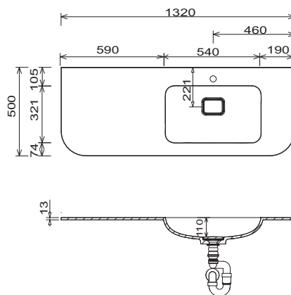
Möbelwaschtisch WMS 263L 61
