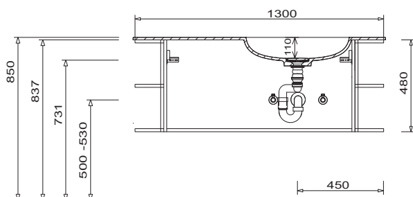
Einzelwaschtisch Ablagefläche links Unterschrankhöhe 480 mm
