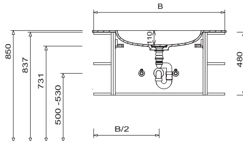
Einzelwaschtisch Unterschrankhöhe 480 mm
