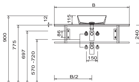
Aufsatzwaschtisch Unterschrankhöhe 240 mm Waschtischhöhe entspricht der Höhe des Nizza rund Waschtisches
