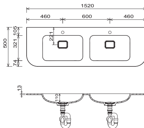
Möbelwaschtisch WMS 263R 61
