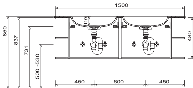
Doppelwaschtisch Unterschrankhöhe 480 mm
