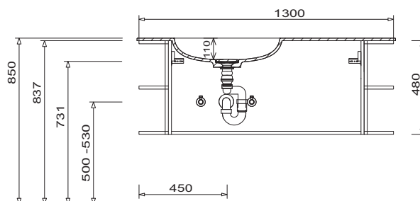
Einzelwaschtisch Ablagefläche rechts Unterschrankhöhe 480 mm
